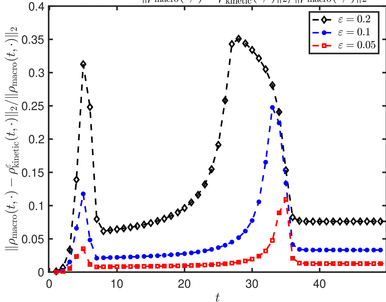
Evolution of \|\rho_{\text{macro}}(t, \cdot) - \rho_{\text{kinetic}}^\varepsilon(t, \cdot)\|_2 / \|\rho_{\text{macro}}(t, \cdot)\|_2
